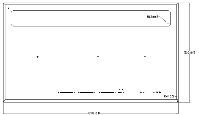
S - DDH2
